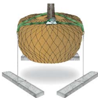
Système d'ancrage: Deadman avec Plati-Mat et Sangle
